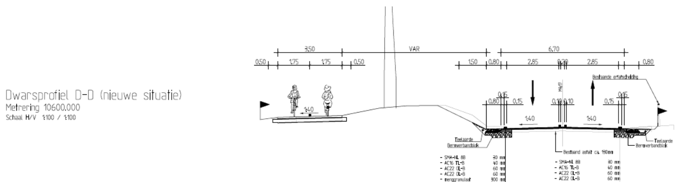
Figuur 3: Dwarsprofiel N417 toekomstige situatie
