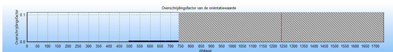
Figuur 8 Overschrijding van het groepsrisico als functie van de stationing van W-533-12 in de toekomstige situatie.
