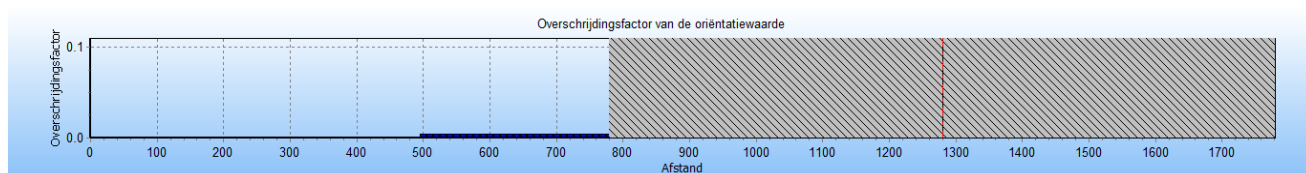
Figuur 6 Overschrijding van het groepsrisico als functie van de stationing van W-533-12 in de huidige situatie.
